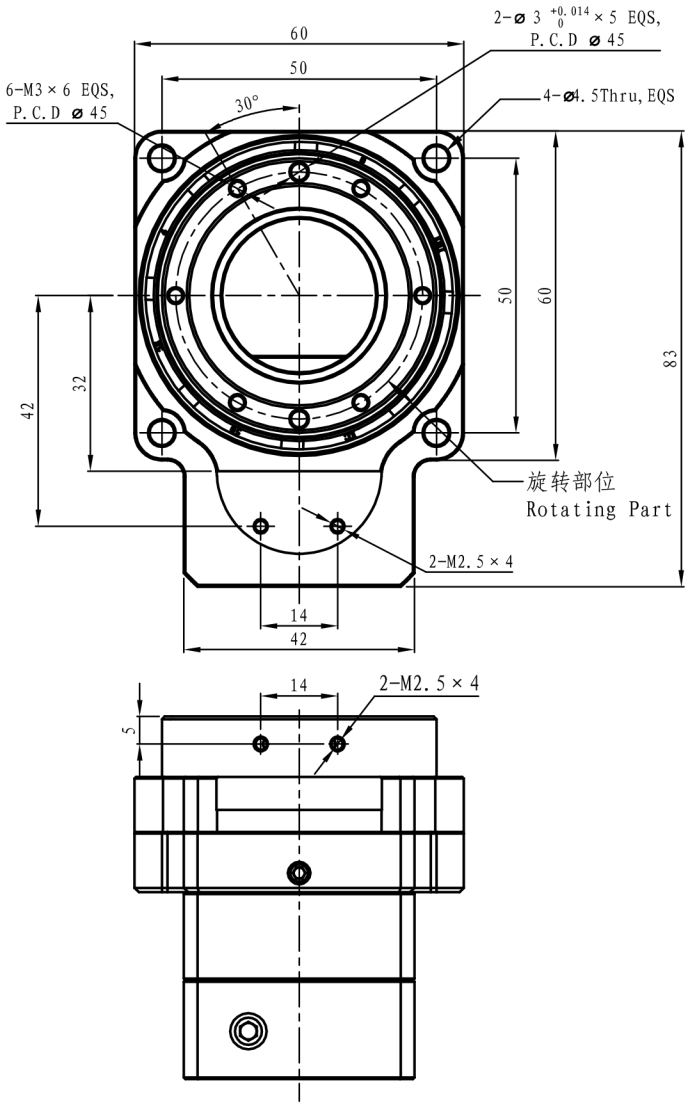
输出端 Output
