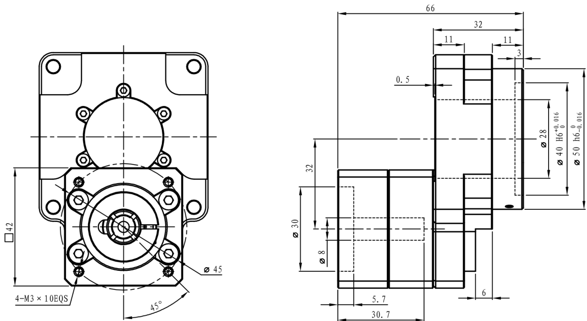
输入端 Input
